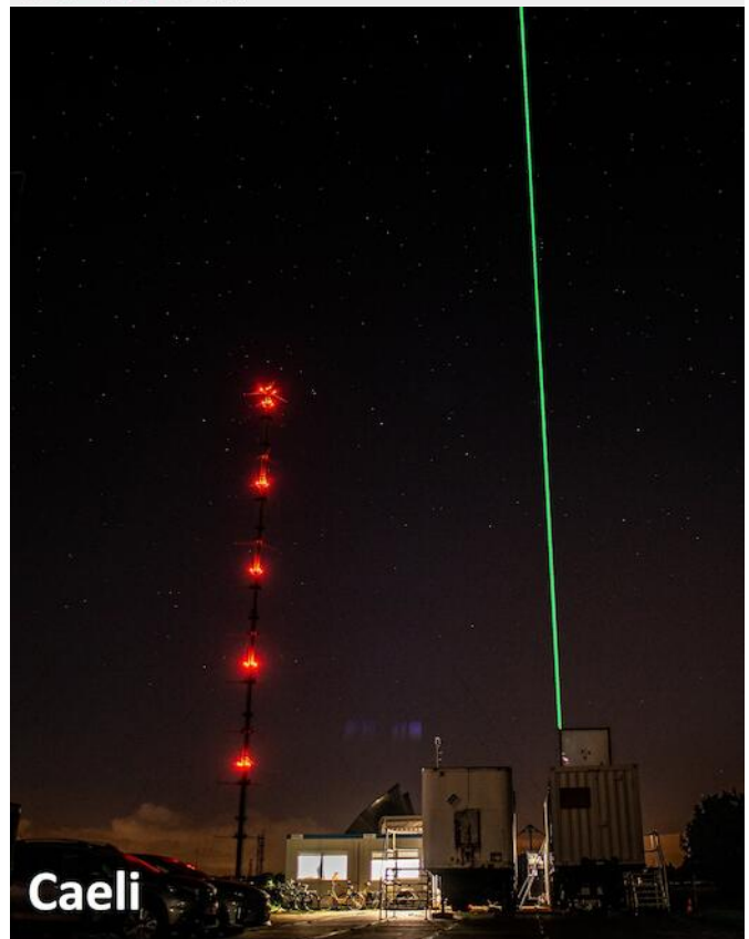
Onderhoud CESAR Water Vapour, Aerosol and Cloud Lidar. Foto: Arnoud Apituley
