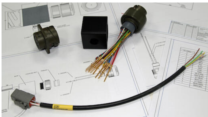
Hybride kabel met power, fiberoptics, ethernet en coax
